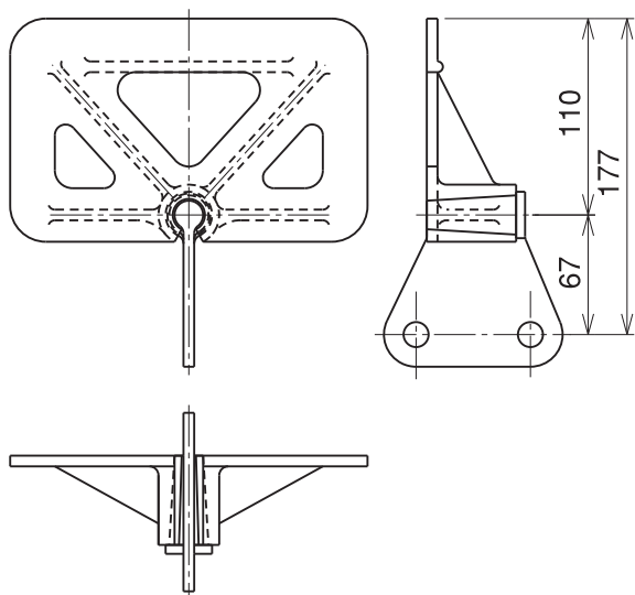
セクショナルサポートMB3
