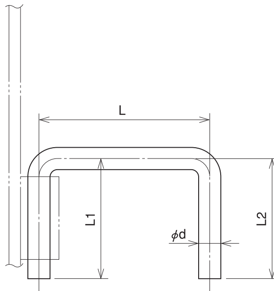
SM3 型式標示 SM3-φ d-L-L1-L2
