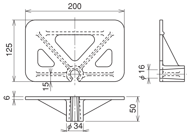
セクショナルサポートMB3
