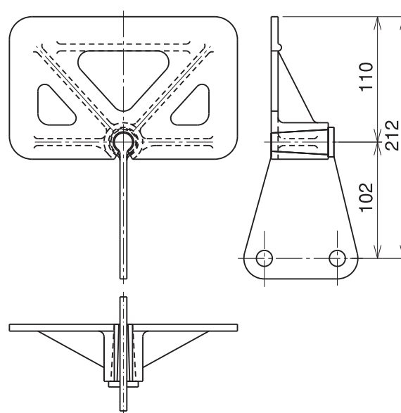
セクショナルサポートMB3N
