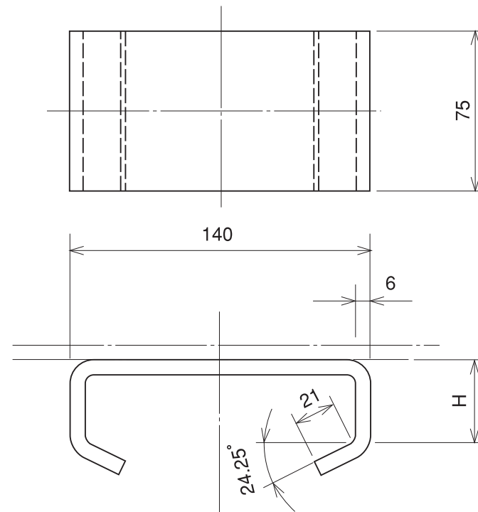
CM2 型式標示 CM2-H
